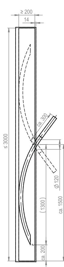
Art. - Nr. 5153 50 - 180
