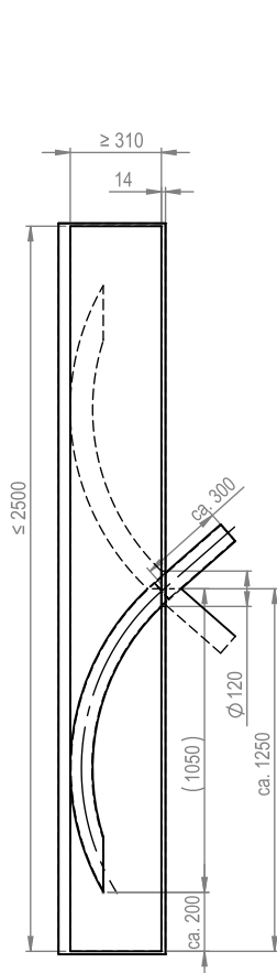
Art. - Nr. 6710 75 - 140
