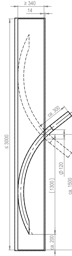
Art. - Nr. 6711 75 - 180
