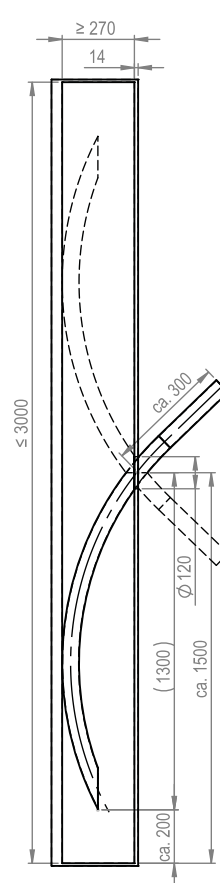
Art. - Nr. 6390 63 - 180
